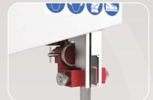
Guidalame superiore e inferiore di alta precisione APA II Guidalame supérieur et inférieur de haut précision APA II High-precision top and bottom blade guide APA II Hochpräzisions obere und obere Blattführung APA II Guía-sierra superior y inferior de alta precisión APA II
